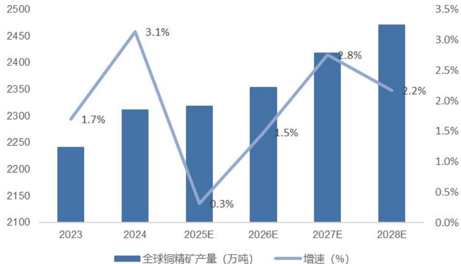
图：全球铜精矿供给及增速
