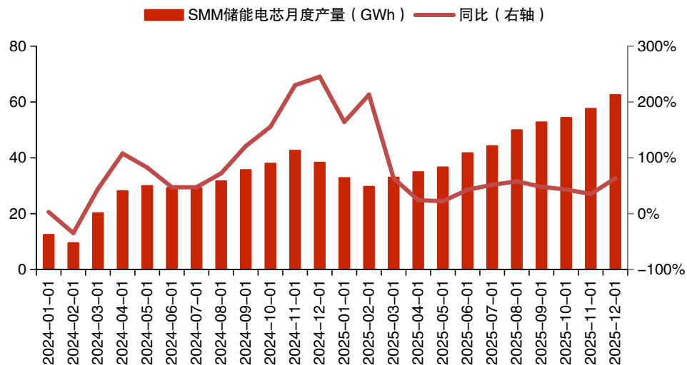
图：储能电芯月度产量
