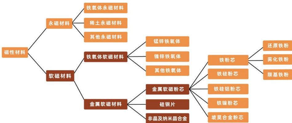
图：软磁材料分类图谱
